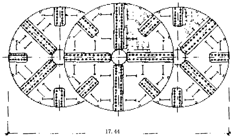
图 员-苑 三圆形盾构
