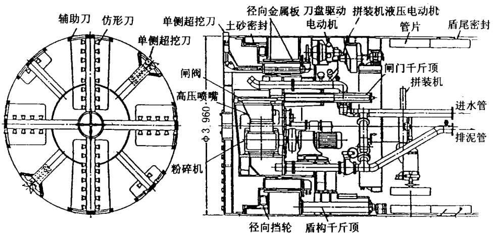
图员猿 泥水盾构
