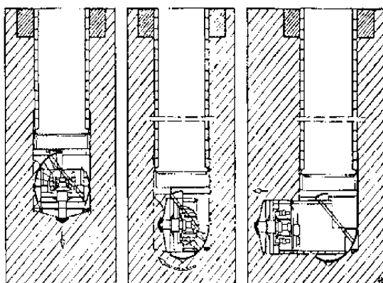
图 员-愿 竖井隧道一体化盾构
