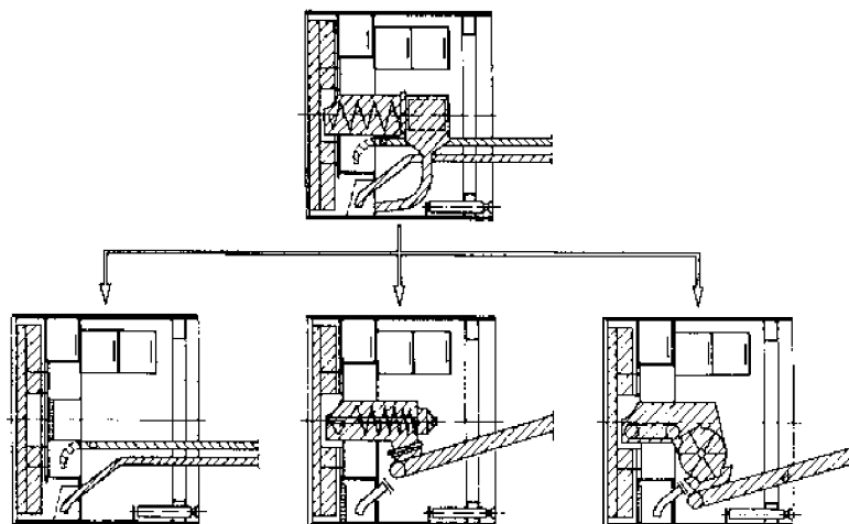
图 1-16 混合盾构
