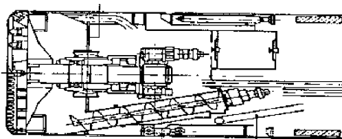
(b) 上压平衡
