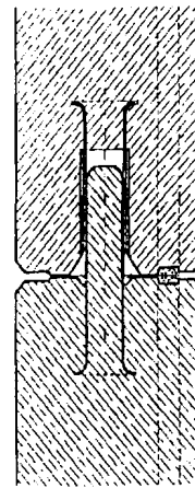
图 1-11 钢销钉
