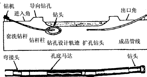
图 员-苑 定向钻进施工法
