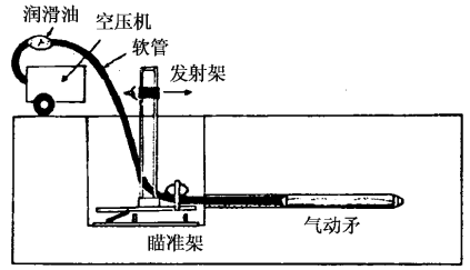
图 员- 缘 气动矛施工法
