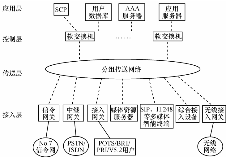
图 2.1 软交换网络结构图
