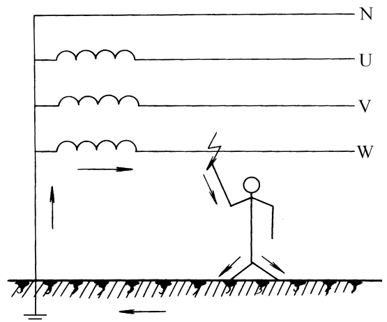
图 1-4 中性点直接接地单相触电
