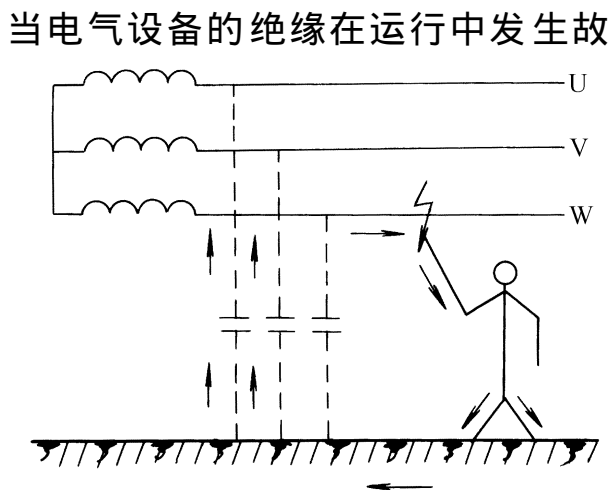
图 1-5 中性点不接地单相触电
