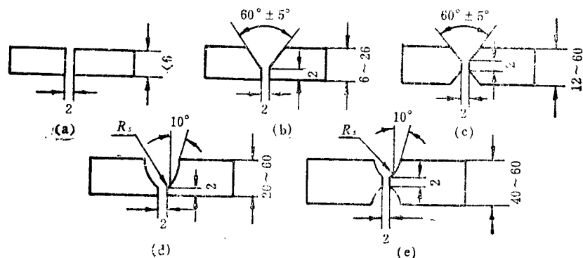
图 1-1 对接接头的坡口型式
