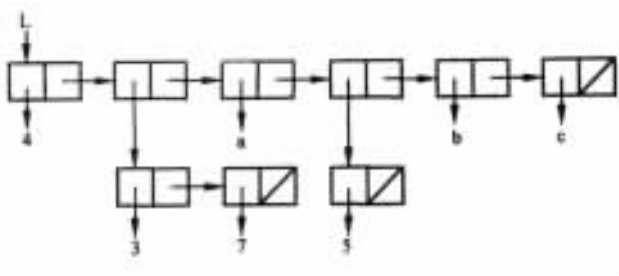
图 2.3 表(4 (3 7) a (5) b c)的链表结构
