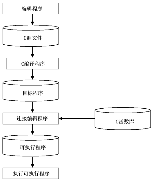
图 1-1 C 语言程序的操作过程
