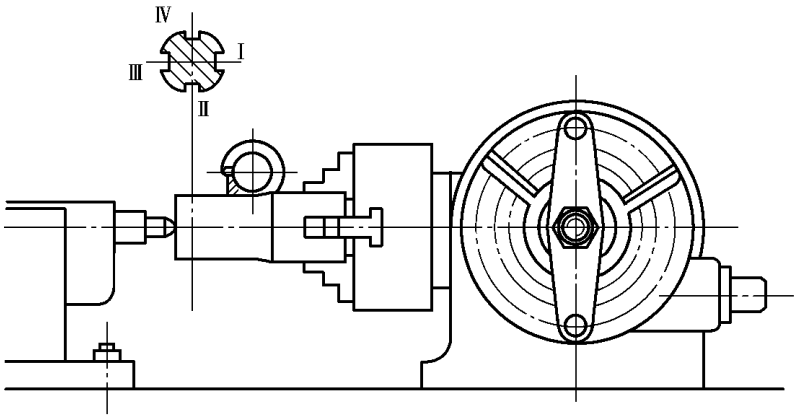
图 员猿 摇多工位加工
