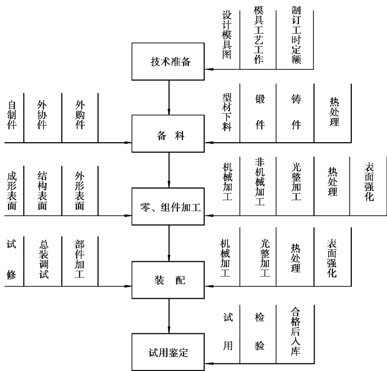
图 1-1 摇模模具的生产过程示意图
