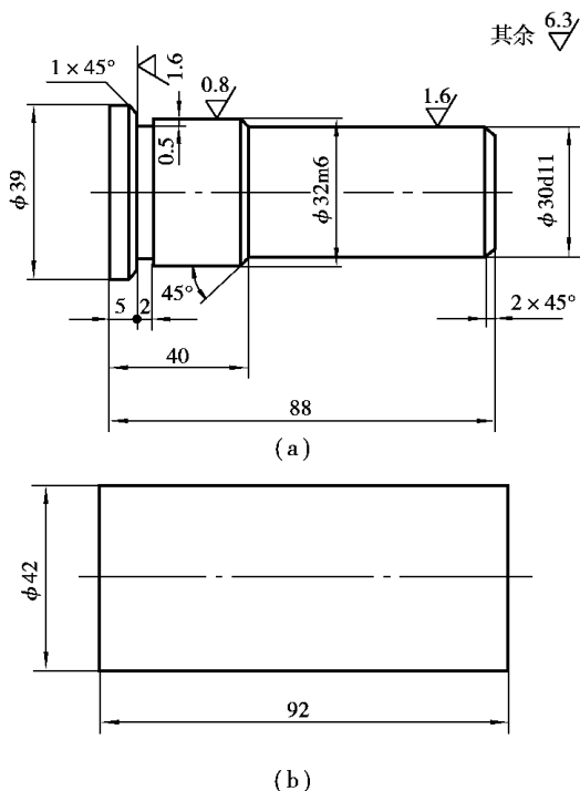
图 1-1 压铸压入式模柄
