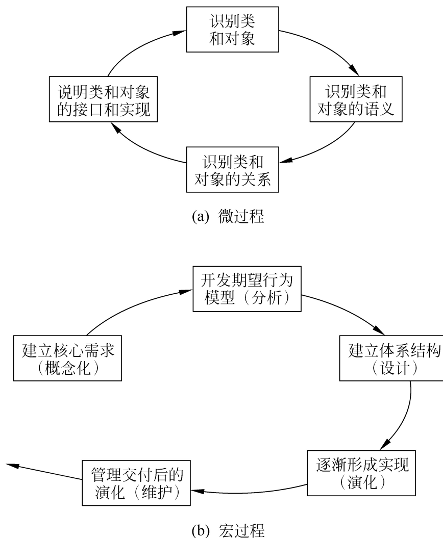
图 1.2 Booch 方法的 OO 开发过程
