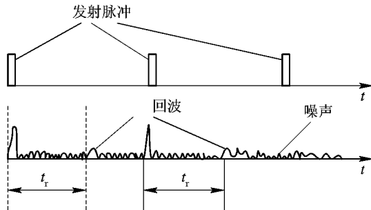
图 1.3 雷达测距
