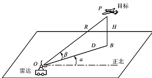
图 1.1 用极(球)坐标系表示目标位置
