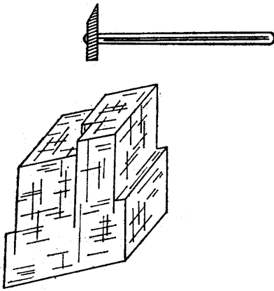
图 1-3 矿物的解理和解理面示意图
