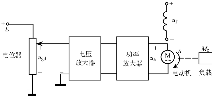
图 1-5 直流电动机转速开环控制系统
