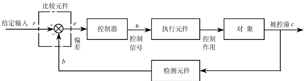
图 1-3 一般自动控制系统框图
