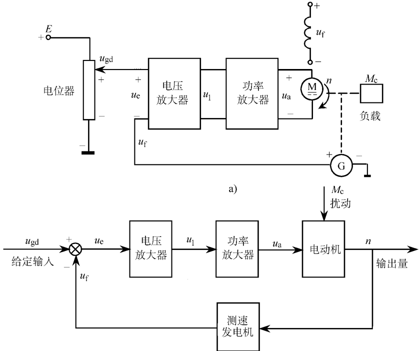
图 1-6 直流电动机转速反馈的闭环控制系统
