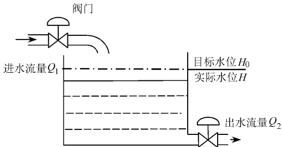
图 1-1 水位人工控制系统示意图
