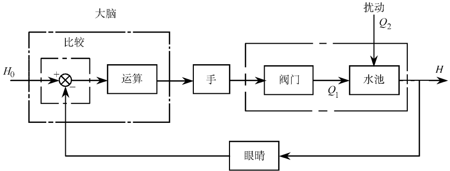
图 1-2 人工水位恒定控制系统原理框图
