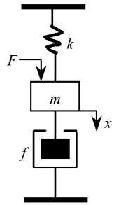
图 2-1 弹簧-质量-阻尼器系统
