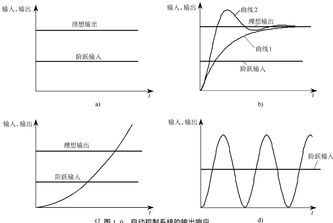
c) 图 1-9 自动控制系统的输出响应
