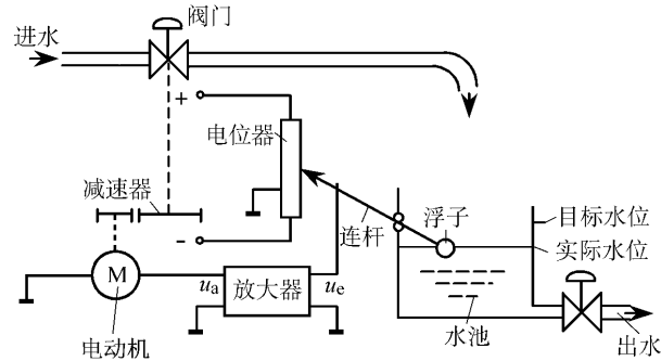
图 1-4 水位自动控制系统
