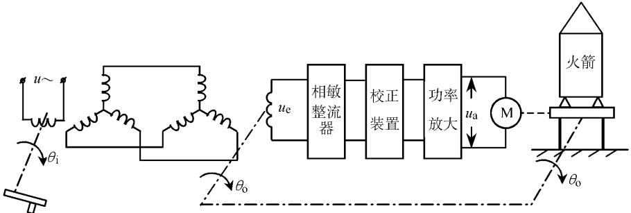
图 1-8 火箭方位角随动控制系统
