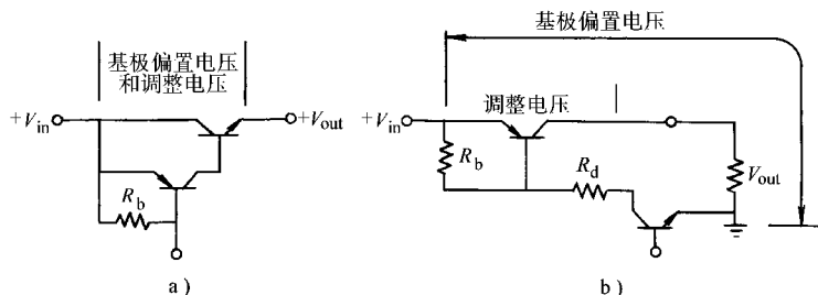
图 4-10 调整管对电压降的影响 a) NPN 调整管 b) PNP 调整管（低电压降）
