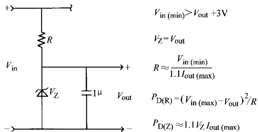
图 10-2 稳压二极管的稳压电路
