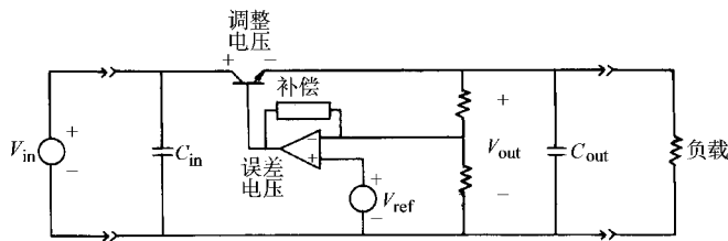
图 10-1 基本线性电源
