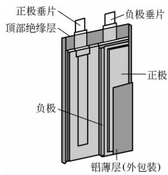
图 1-6 聚合物锂离子电池的几种结构
