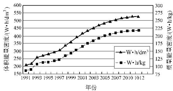
图 1-5 聚合物锂离子电池的能量密度发展趋势
