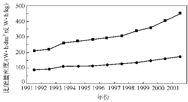
图 1-2 18650 型锂离子电池的能量密度发展趋势
