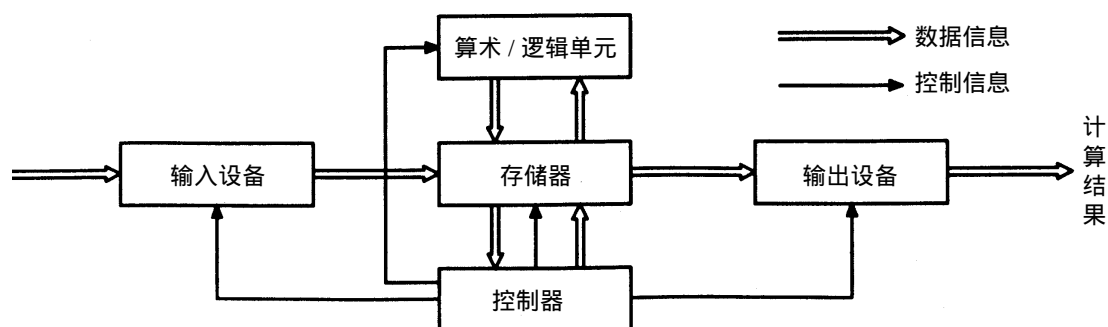
图 1.1 冯·诺依曼计算机硬件结构
