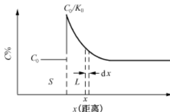
图 2-2-2 稳定生长中溶质的再分布
