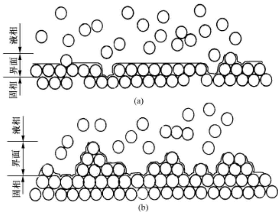
图 2-1-2 固液界面的微观形貌
