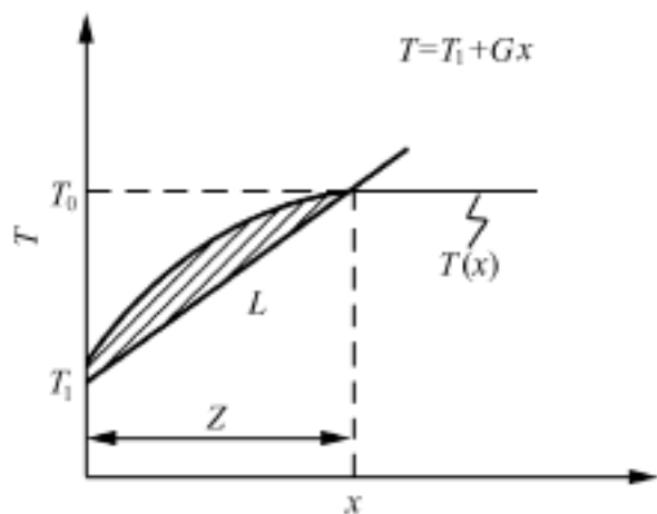
图 2-2-3 成分过冷示意图
