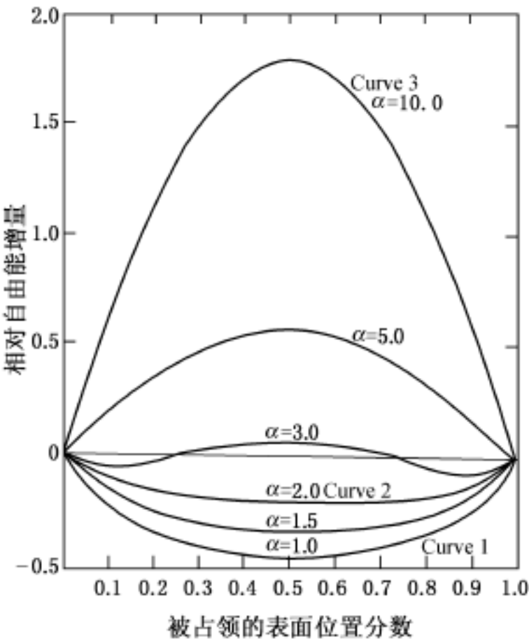
图 2-1-1 表面相对自由能增量与被占领的表面位置分数的关系曲线 (Jackson [13] )
