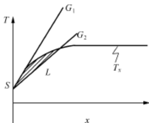
图 2-3-1 成分过冷示意图
