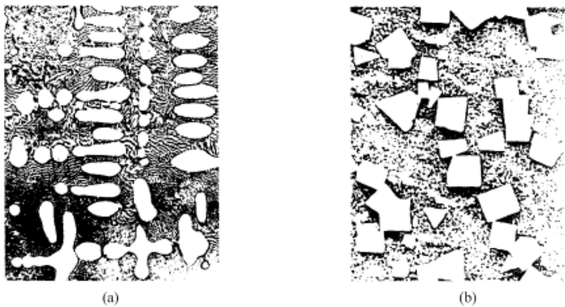
图 2-1-4 金属系的固液界面结构
