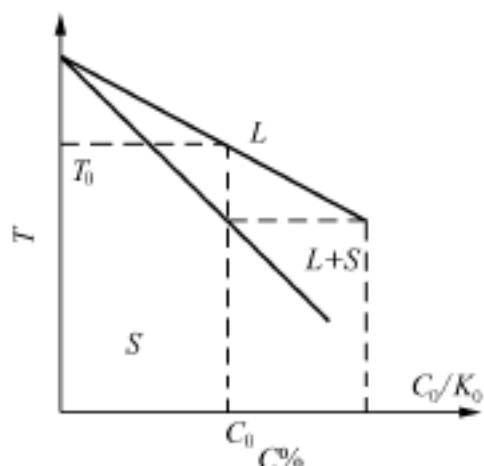
图 2-2-1 平衡相图一角
