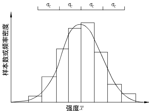
图 1 材料强度正态分布曲线
