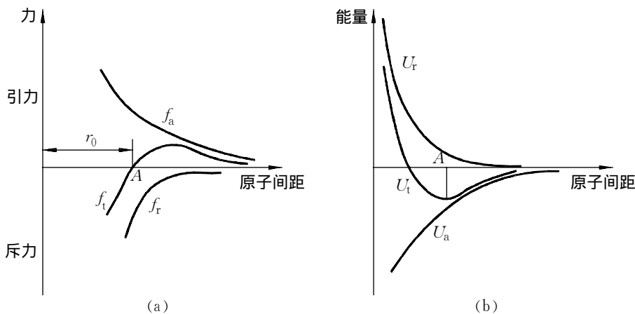
图 1-1 物质内部质点相互作用的力、能量与质点间的关系 (a) 作用力(力)与原子间距(距离)的关系 (b) 能量(能)与原子间距(距离)的关系
