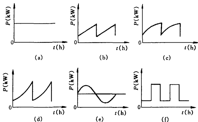
图 2-1 生产机械的典型负荷曲线
