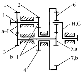
图 2-2 封闭行星轮系机构
