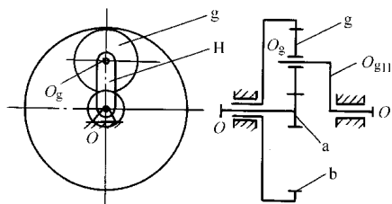
图 1-1 周转轮系
