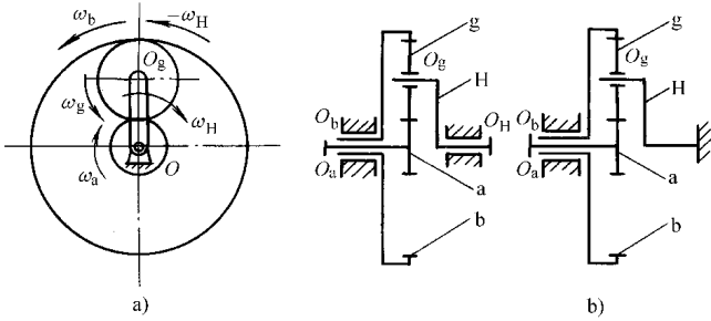
图 2-1 行星齿轮传动及其转化机构
