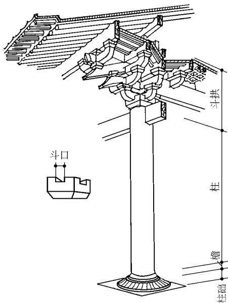
图 1-1-1 木斗拱结构
