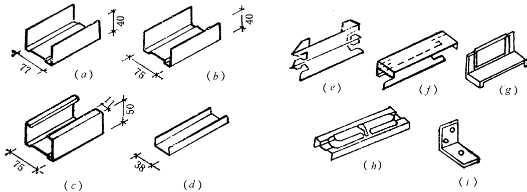
图 猿猿猿猿 悦核系列龙骨主件和配件示意
