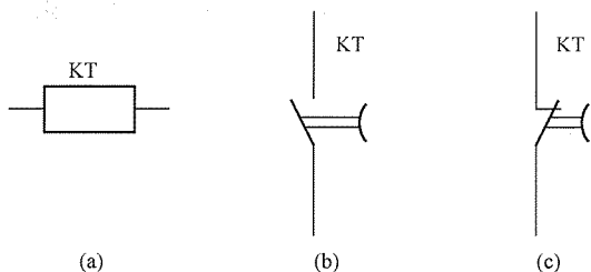
图 1-3 时间继电器结构
