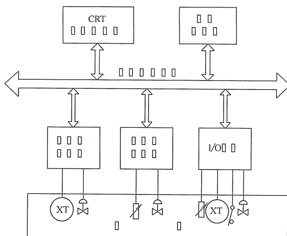
图 1-21 集散控制系统基本组成框图
