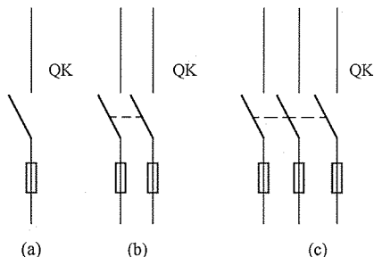
图 1-6 刀开关
