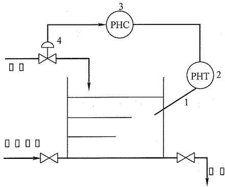
图 1-18 PH 控制系统
