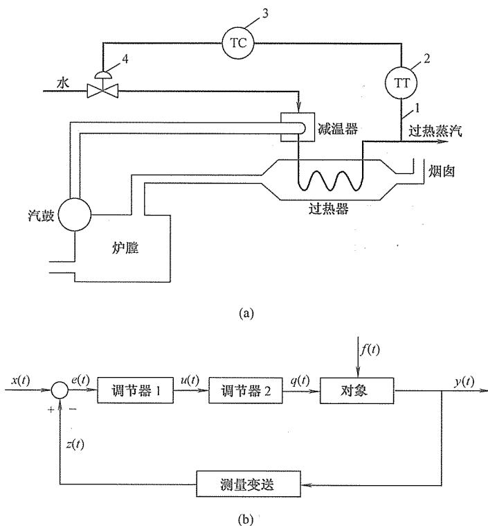
图 1-17 过热蒸汽温度控制系统
