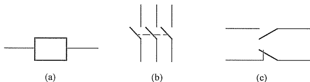
图 1-1 接触器结构
