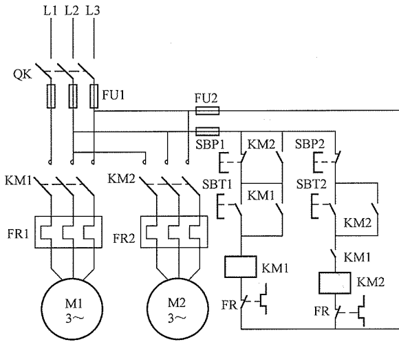
图 1-10 顺序控制电路
