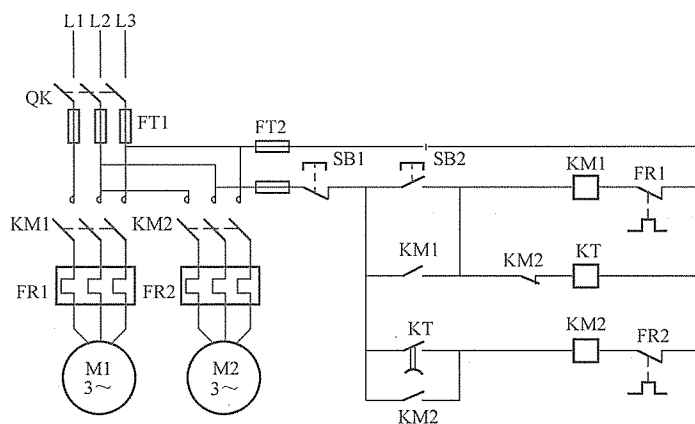
图 1-12 定时控制
