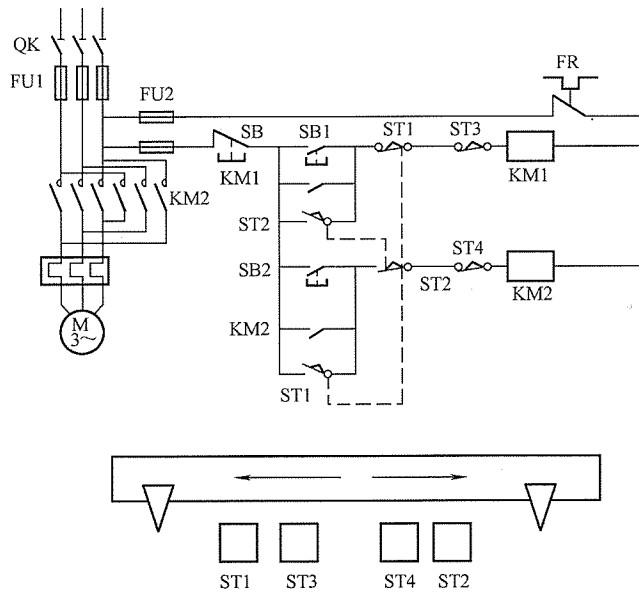
图 1-11 行程控制
