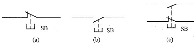
图 1-7 按钮电气符号
