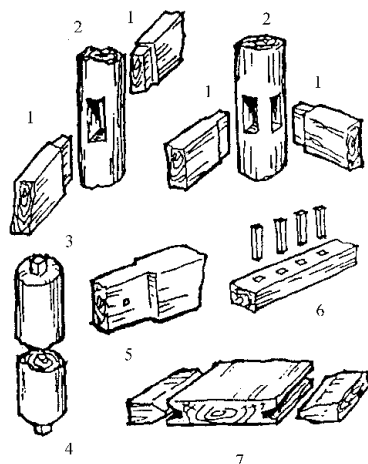
图员-员-源河姆渡遗址木构件 员-梁摇圆-柱摇猿-柱头榫摇源-柱脚榫 缘-有钉孔的梁头榫摇远-栏杆榫卯摇苑-企口板
