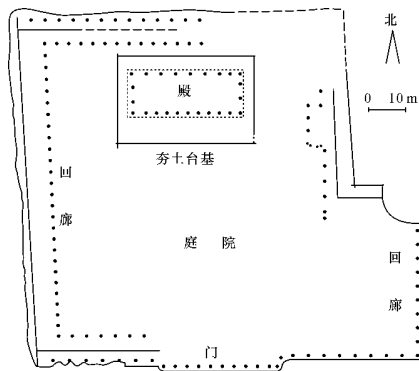
图员-员-缘河南偃师二里头宫殿遗址
