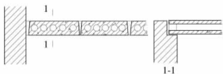
图 2-10 预制空心板
