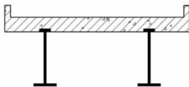
图 2-2 钢-钢筋混凝土组合梁
