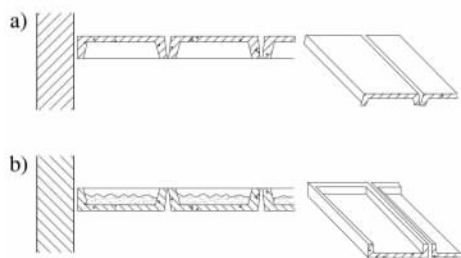
图 2-9 槽形板
