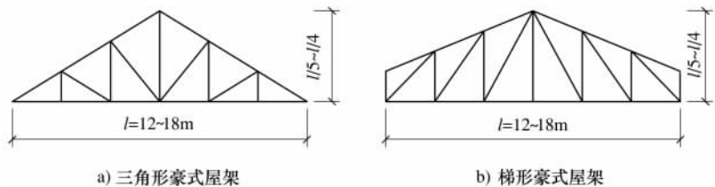
图 3-3 豪式木屋架
