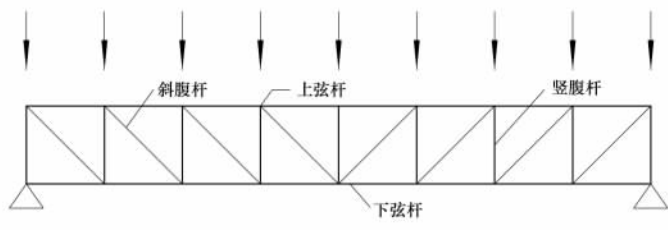
图 3-1 桁架示意
