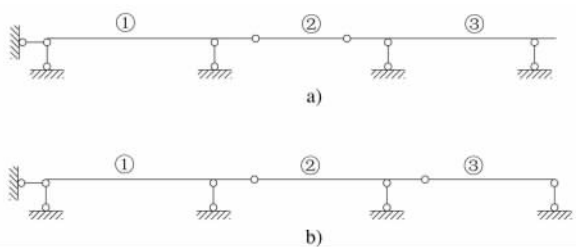
图 2-6 三跨静定梁
