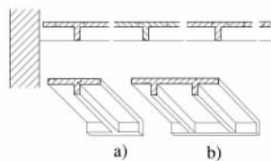
图 2-11 T 形板
