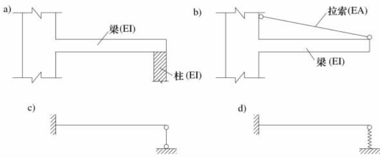
图 2-5 悬臂端设支柱或拉索的悬挑梁
