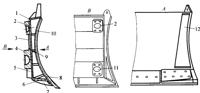
图 1-5 推土刀的构造
