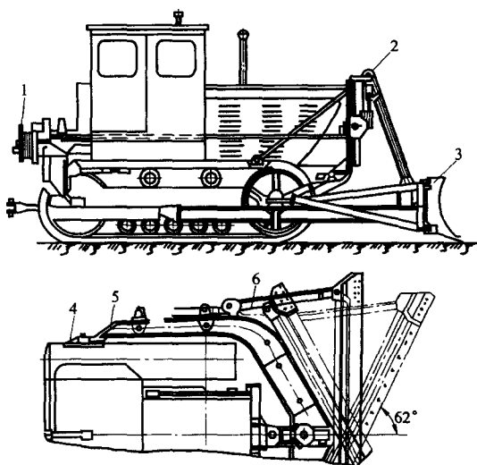
图 1-2 回转式推土机（斜铲）
