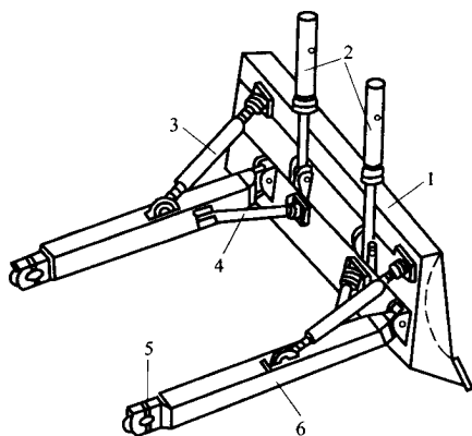
图 1-6 固定式推土机工作机构
