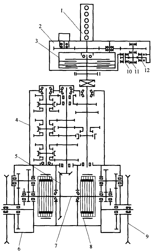
图 1-4 液压操纵履带式推土机底盘传动图 1—发动机；2—齿轮箱；3—主离合器；4—变速箱； 5—中央传动室；6—最终传动装置；7—横向分配轴； 8—转向离合器；9—链轮；10—主离合器泵驱动轴； 11—转向离合器泵驱动轴；12—工作装置油泵驱动轴
