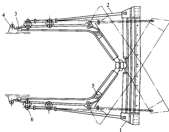
图 1-7 回转式推土机工作机构
