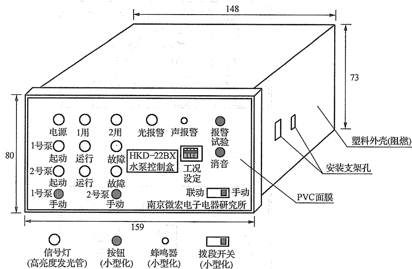
两台水泵控制盒外观示意图
