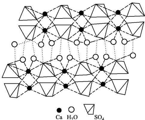
图 员猿 二水石膏的结晶结构
