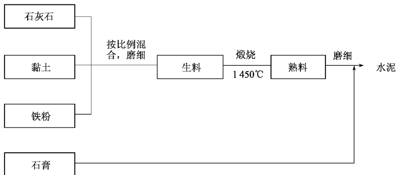
图员员 硅酸盐水泥生产工艺流程
