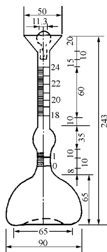
图 1-1-1 李氏瓶
