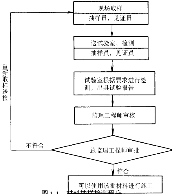
图 1-1 材料抽样检测程序
