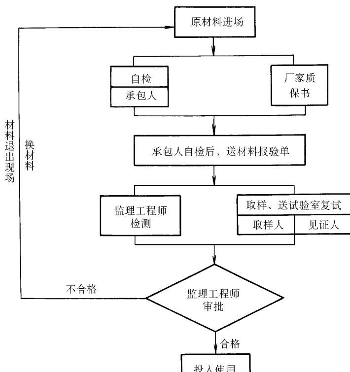
图 1-2 原材料质量监理工作程序
