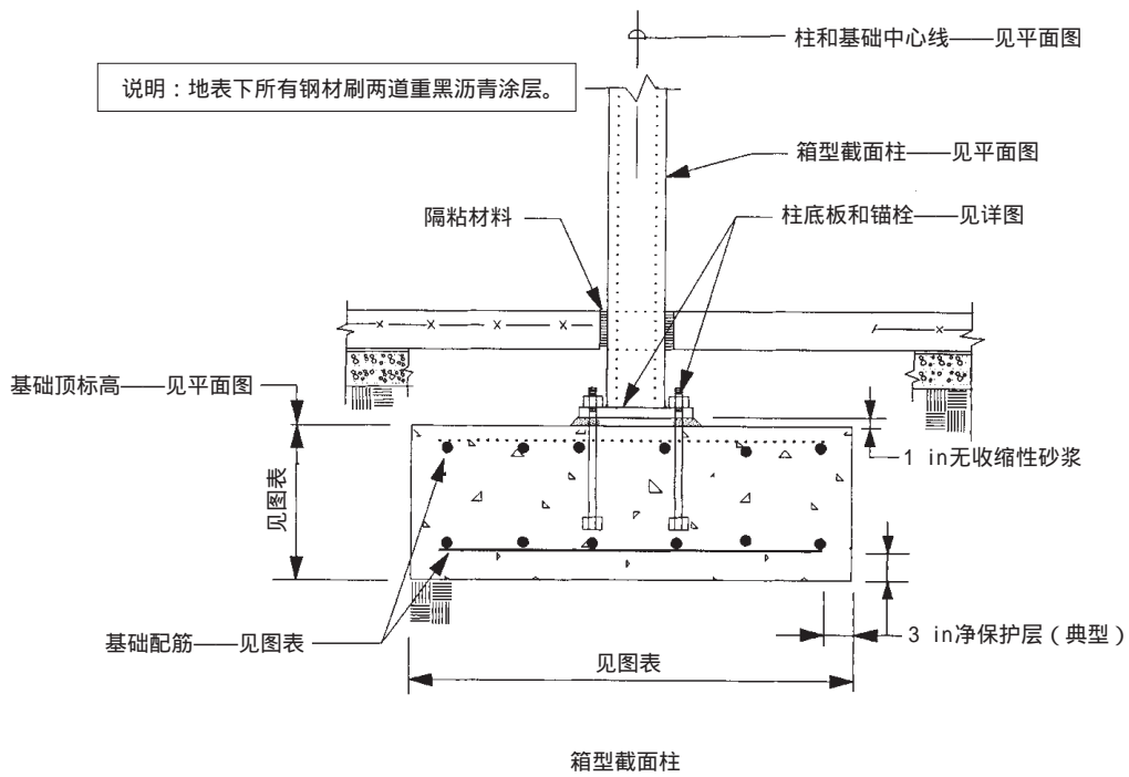
典型内柱 / 基础详图 #2
