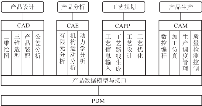
图 1-3 CAD/CAE/CAPP/CAM 系统功能与数据管理
