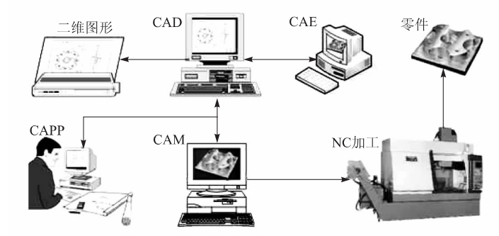
图 1-2 CAD/CAM 在制造过程中的信息流程
