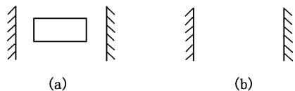
图 1.1 开放式光学谐振腔 (a) 有源腔; (b) 无源腔
