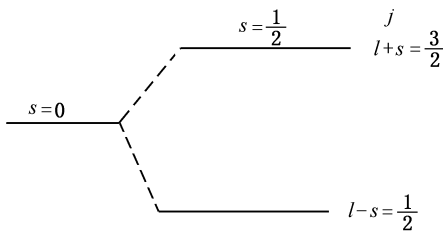
图 10-1 自旋的存在引起能级的分裂
