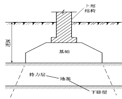
图 1-1 地基基础示意图
