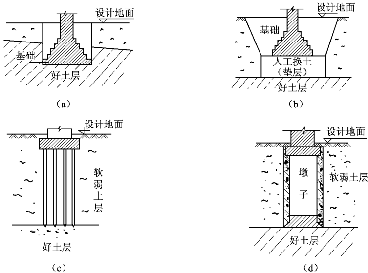
图 1 天然地基基础类型
