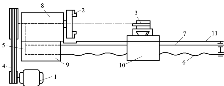
图 员源 普通车床组成的示意图
