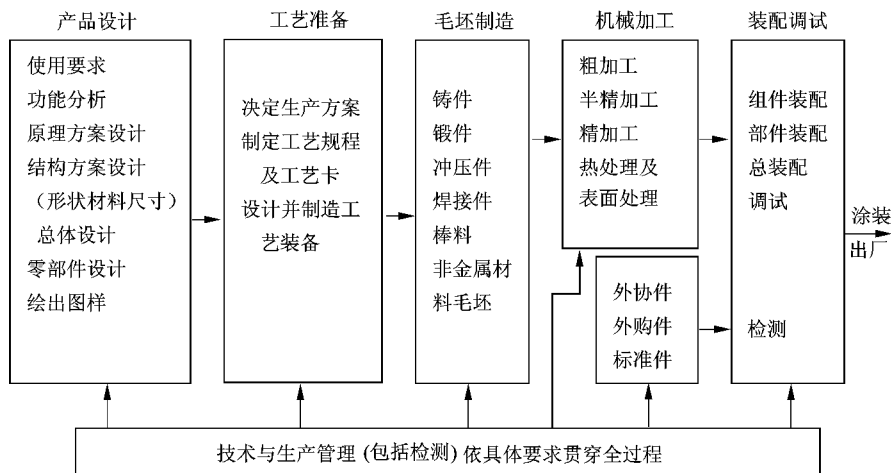
图 1-1 机械产品生产过程
