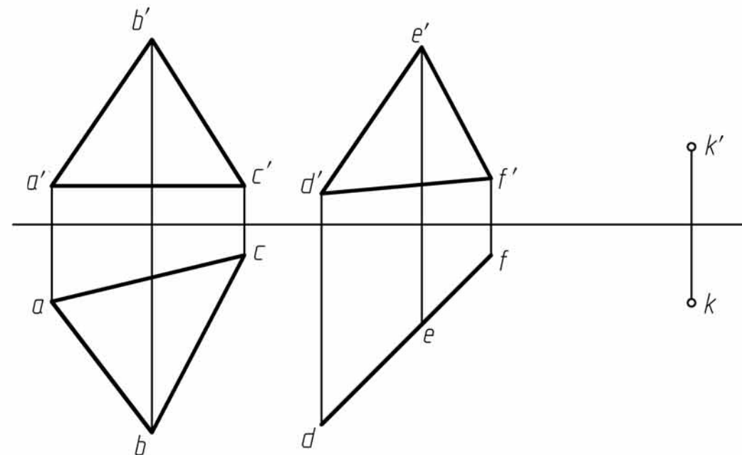
2-26 过点K作直线KM平行于 \triangle ABC 和 \triangle DEF 。
