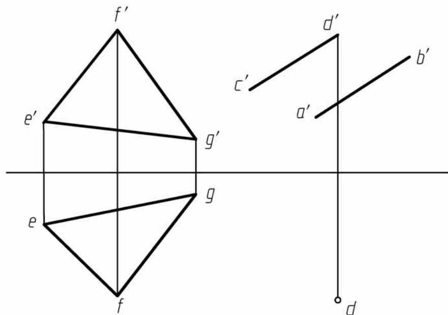
2-27 已知直线AB和CD( AB \parallel CD )所确定的平面平行于 \triangle EFG , 完成该平面的水平投影。
