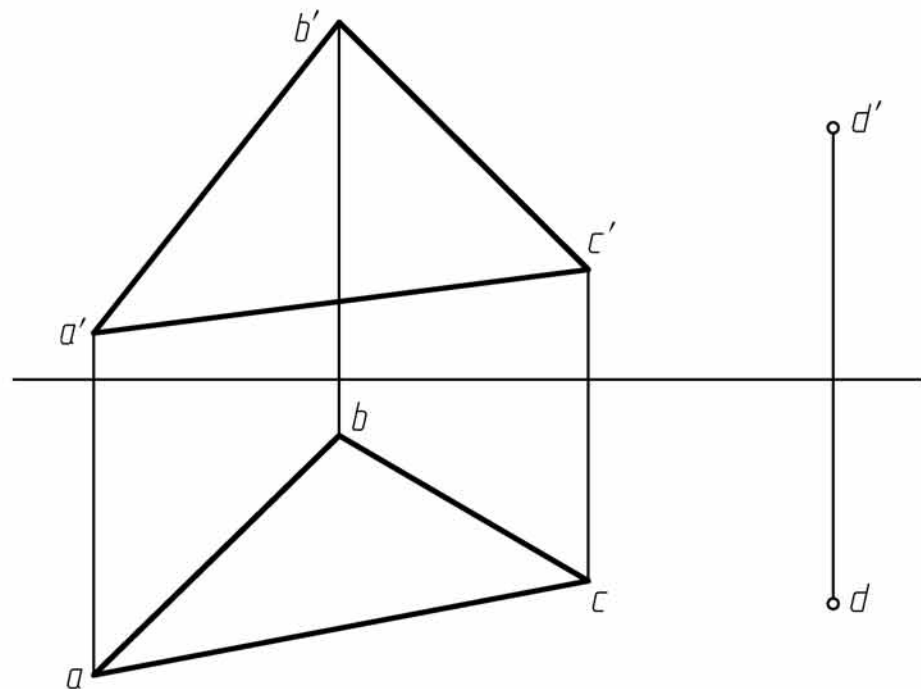
2-25 过点D作正平线DE与 \triangle ABC 平行。
