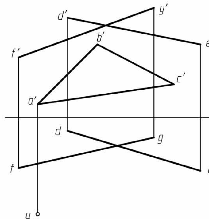
2-28 \triangle ABC 平行于直线DE和FG, 补全 \triangle ABC 的水平投影。
