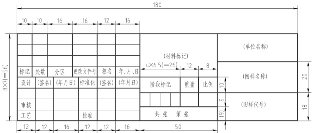
图 1-8 标题栏的格式及尺寸 (参考画法)
