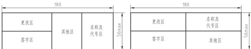
图 1-7 标题栏的组成
