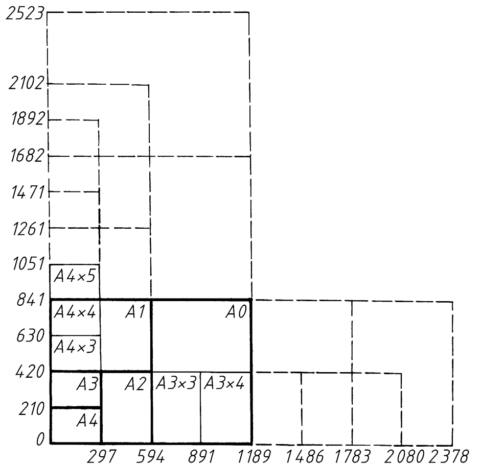
图 1 - 1 基本幅面与加长幅面
