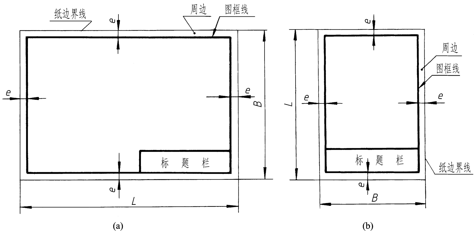
图 1 - 2 不留装订边的图框格式
