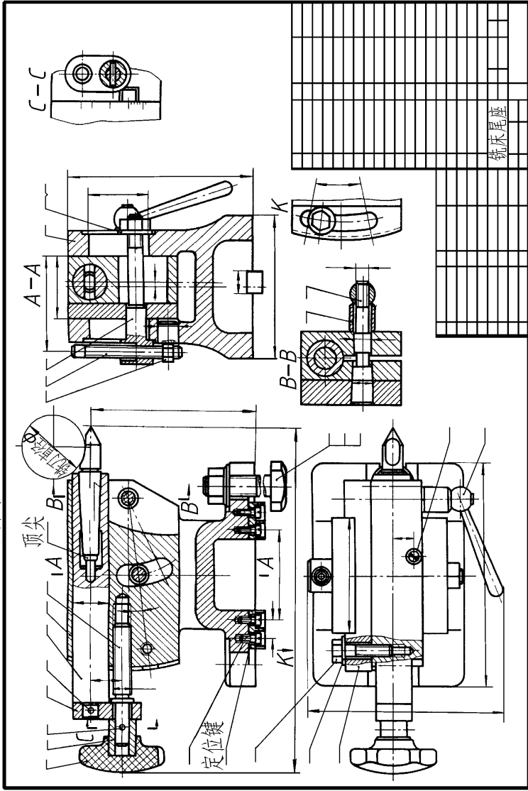
部件装配图 (铣床尾座)
