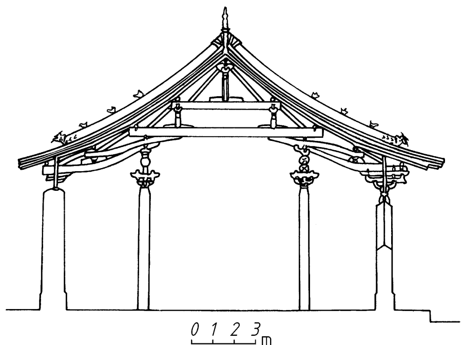
图 0-2 广胜下寺大殿木结构
