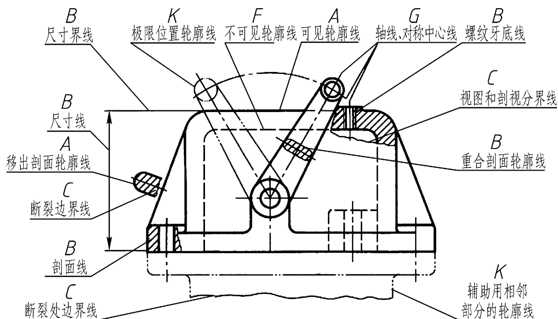
图 1 - 8 图线画法示例
