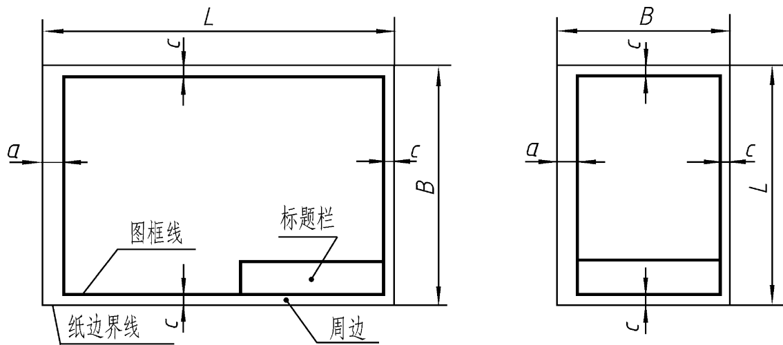
图 1 - 1 留有装订边图样的图框格式
