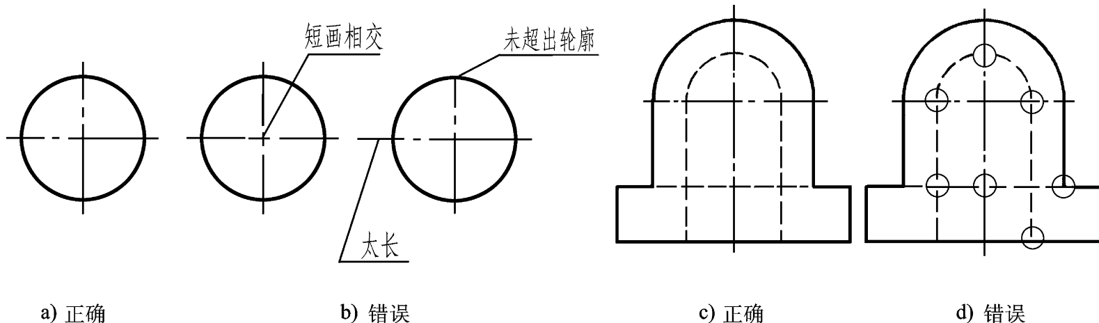
图 1 - 7 点画线、虚线与虚线、虚线与粗实线相交画法
