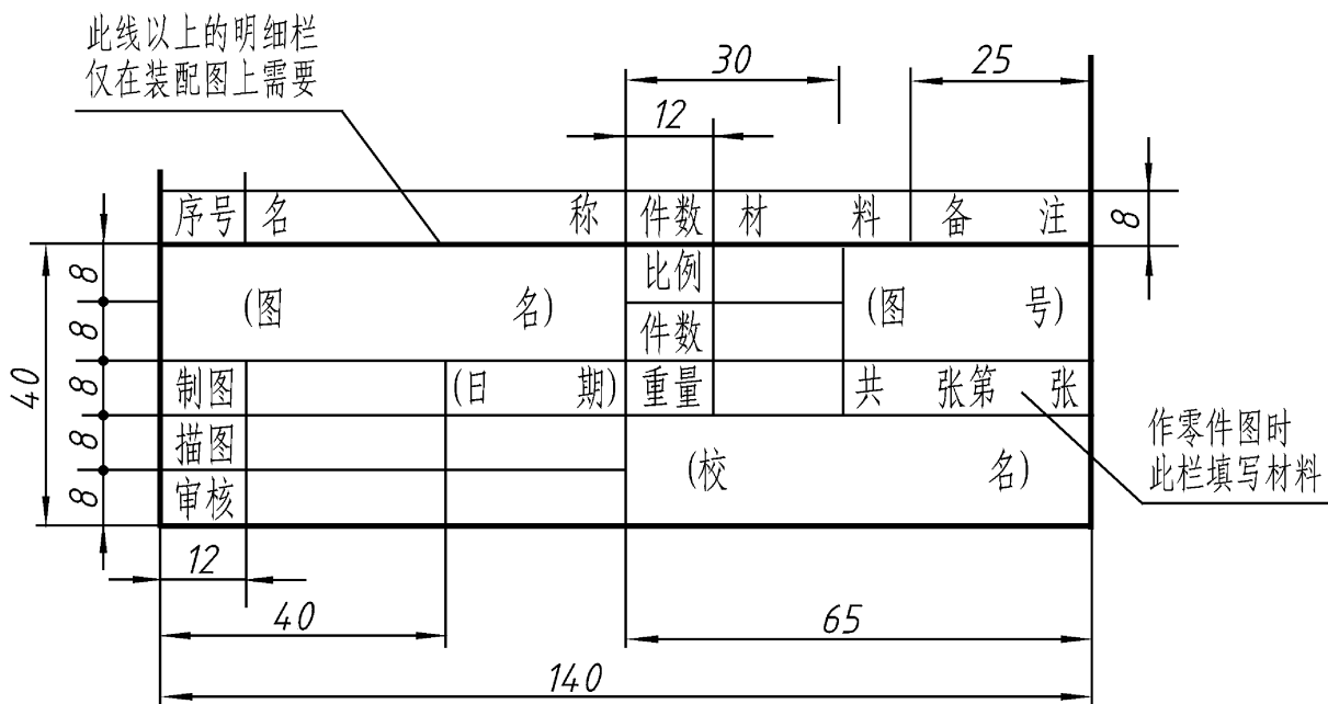
图 1 - 3 制图作业标题栏
