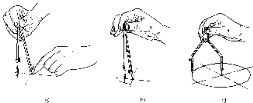
图 1-19 圆规的使用 葬 将针尖扎入圆心 遭 圆规向划线方向倾斜 糟 画大圆时圆规两脚垂直纸面
