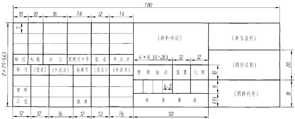
图 员原远 标题栏格式、分栏及尺寸
