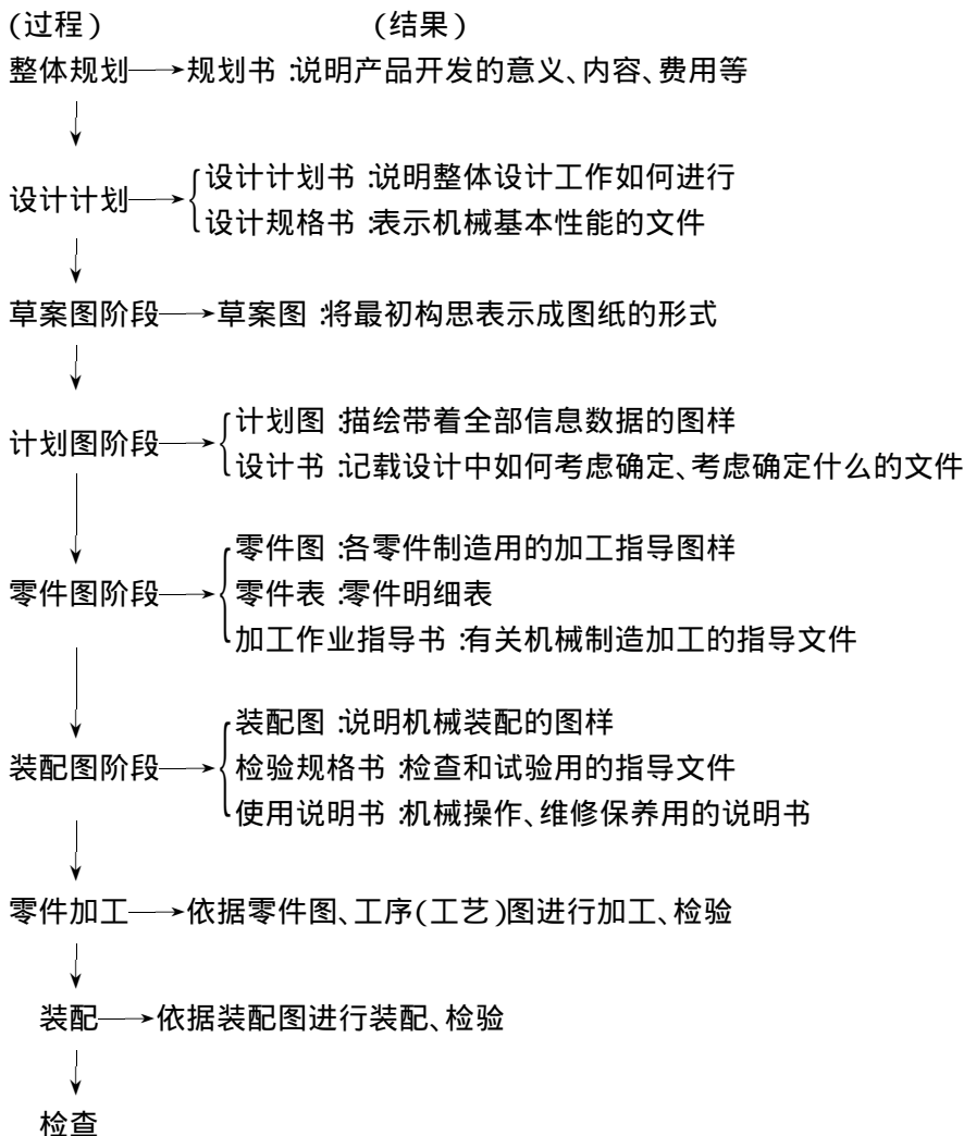
图 园原员 机械设计与制造的过程及结果
