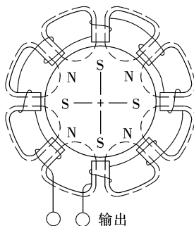
图 1-1-2 发电机式转角计工作原理
