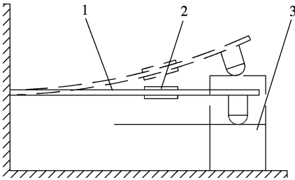
图 1-1-10 电阻应变式测微仪结构原理 弹性悬臂梁 电阻应变片 待测物体
