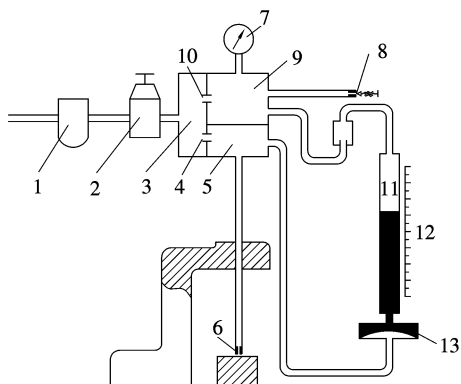
图 员圆 摇典型气动量仪的工作原理
