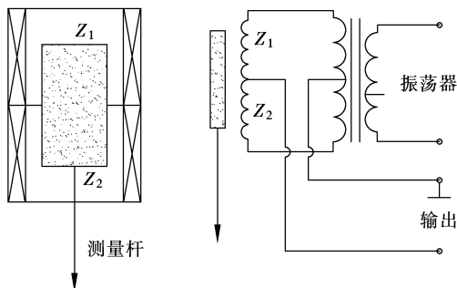
图 1-10 电感式传感器原理及电路
