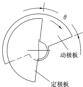
图 1-1-1 电容式角度和角位移测量仪工作原理
