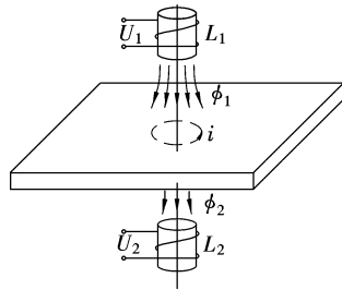
图 1-1-11 涡流式测微仪 结构原理
