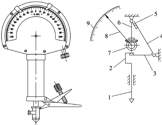
图 圆摇杠杆式齿轮比较仪外形及传动原理
