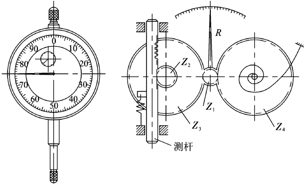
图 圆摇百分表及其传动原理
