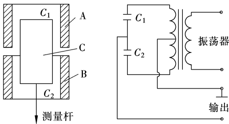
图 1-1-12 变面积型电容式传感器原理及电路
