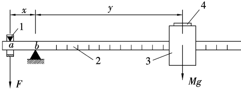
图 员 摇动机械式测量力
