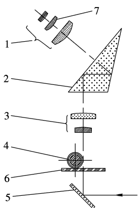
图 员圆 摇测量显微镜 工作原理
