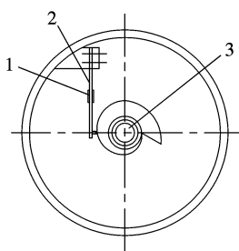
图员圆圆摇应变计式角位移测量仪原理 员是应变片摇圆是悬臂梁摇猿是旋转轴
