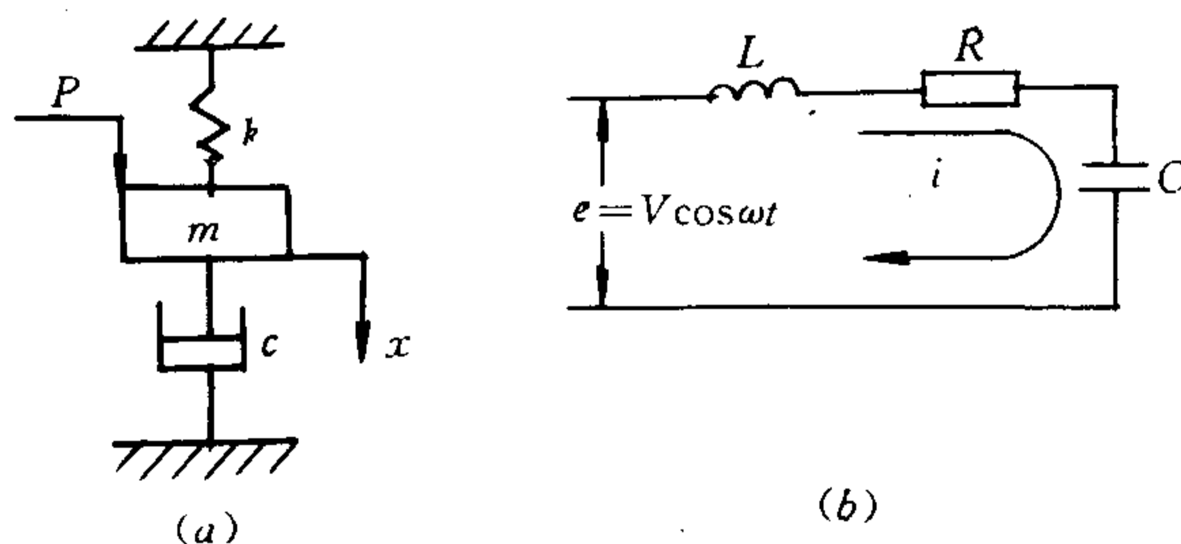
图 1-1 力-电压相似原理
