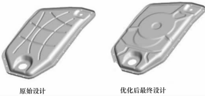
图 1 原形结构的拓扑优化设计结果比较
