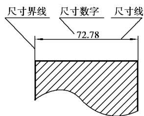
图 1-1-2 尺寸的构成
