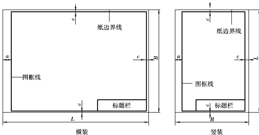
图 1-1-1 留装订边的图框格式
