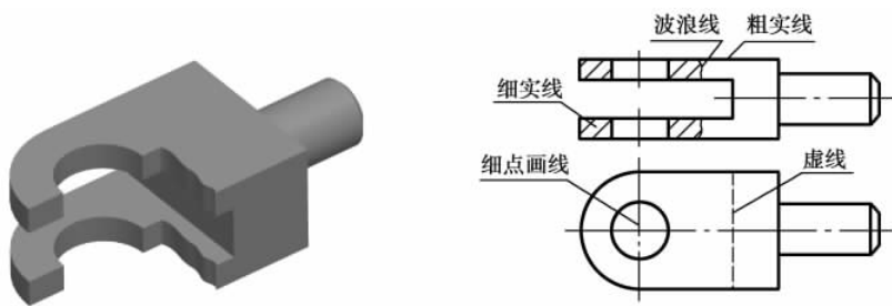
图 1-1-1 图线的应用实例
