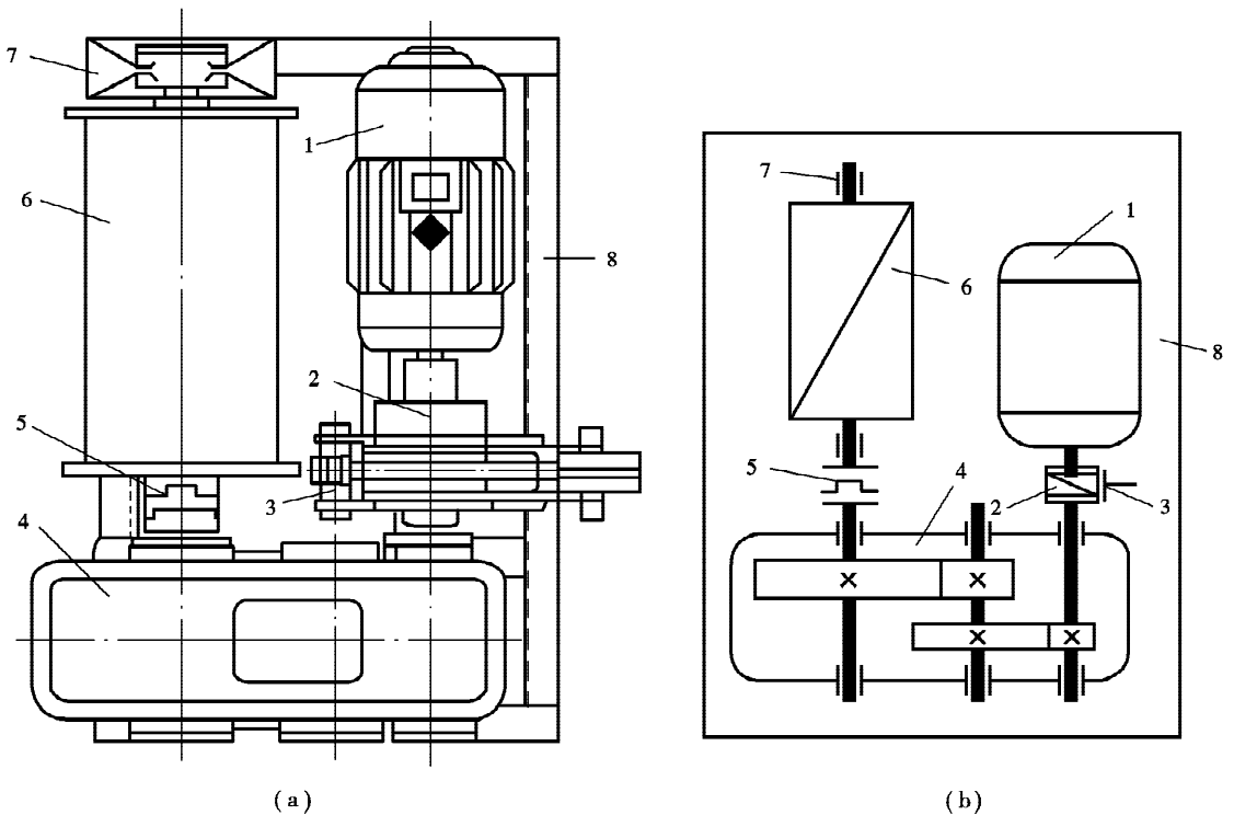
图 员-电动机 圆缘-联轴器 猿-制动器 源-减速器 远-卷筒 苑-滚动轴承 愿-机架 图 员-手摇电动绞车
