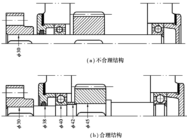
图 1-10 轴的结构
