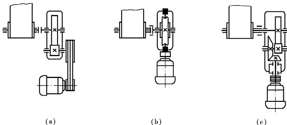
图 8-1 带式运输机的三种传动方案
