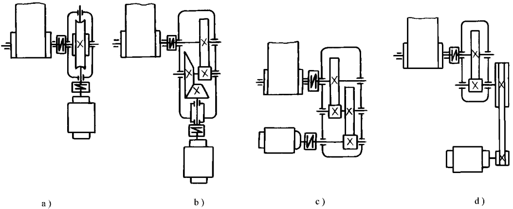
图 2-3 带式运输机的四种传动方案
