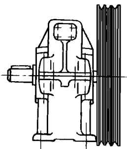
图 2-4 带轮与地基相碰
