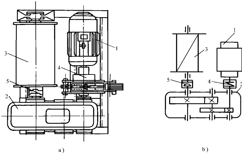
图 2-2 电动绞车及其传动简图
