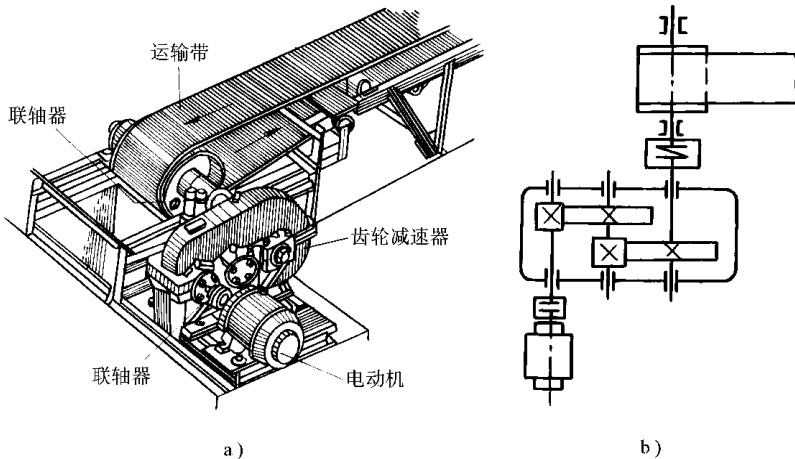
图 2-1 带式输送机及其传动简图
