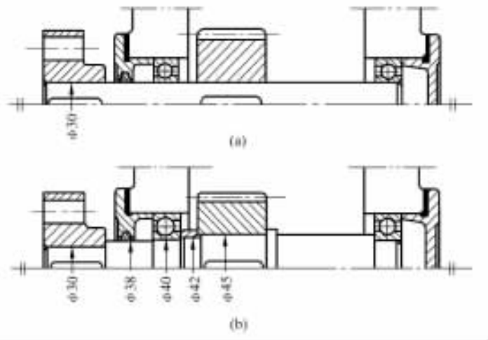
图 1-1 轴的结构设计
