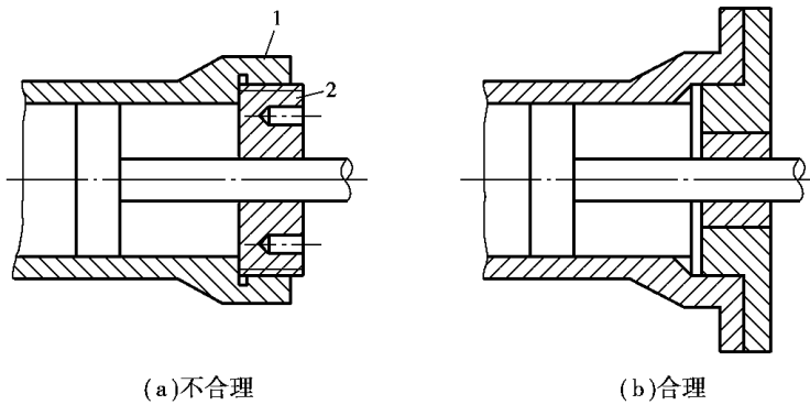
图 1-15 不应以螺纹面对中
