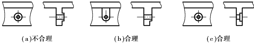
图 1-17 避免采用活块
