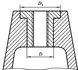
图 1-1-12 减少不必要的配合面
