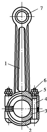
图 1-1 内燃机连杆
