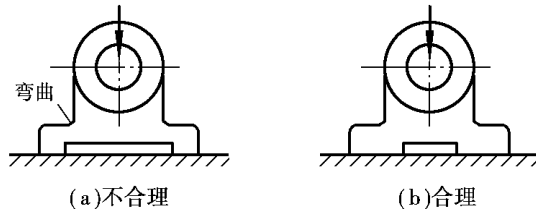
图 1-18 避免铸铁受拉力
