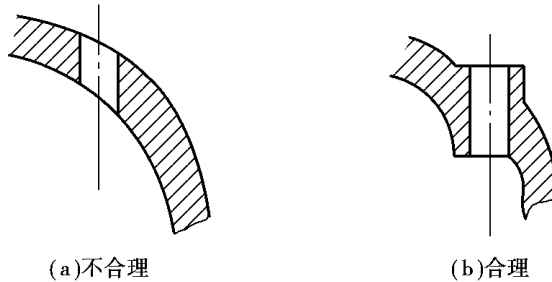
图 1-1-13 避免在斜面上钻孔
