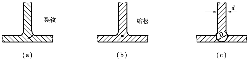
图 1-15 铸件过渡圆角大小应当适当
