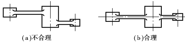
图 1-16 铸件应有明显的分型面
