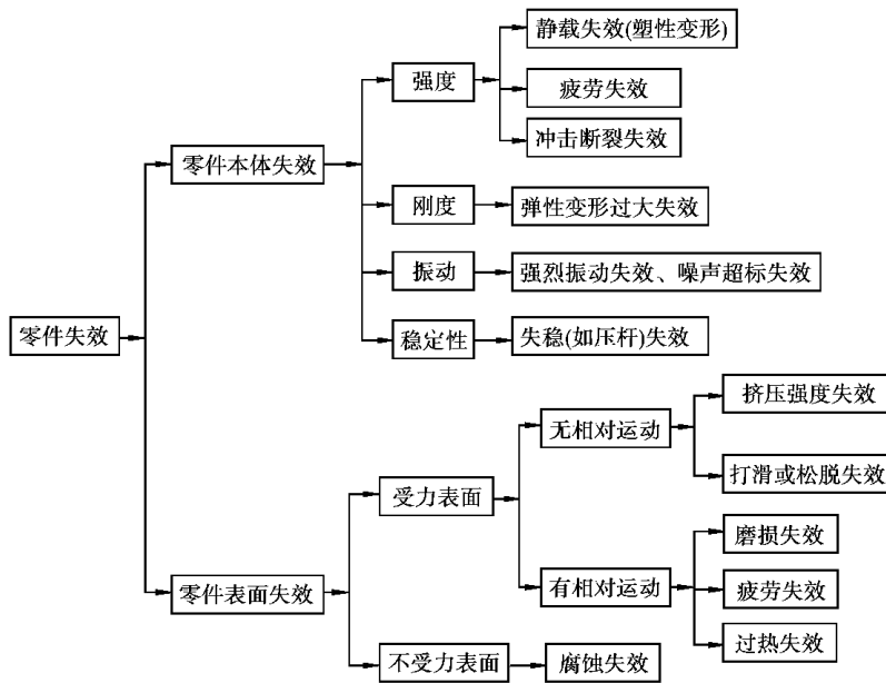
图 1-1 机械零件失效形式框图
