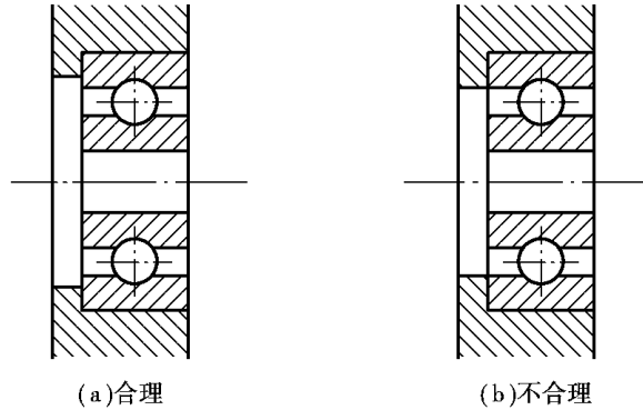
图 1-16 应使拆卸方便
