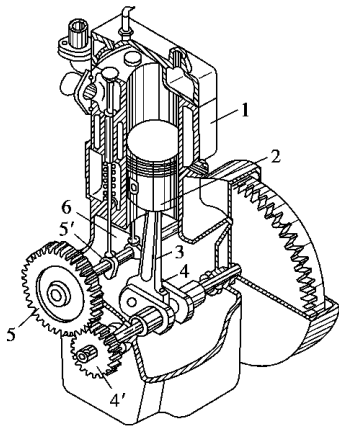
图 员圆猿 内燃机
