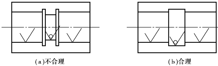
图 1-1-11 二孔在一次安装中加工
