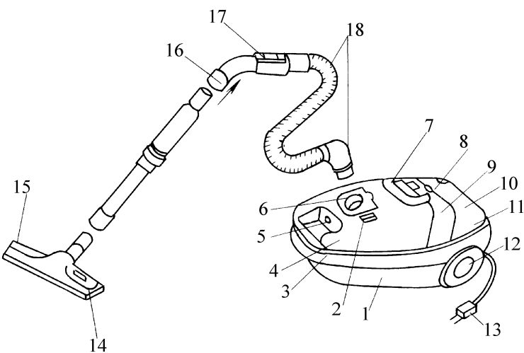
图 1-3 家用吸尘器
