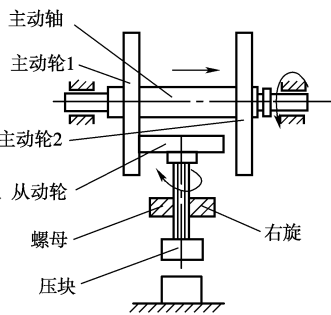
图 1-25 摩擦压力机
