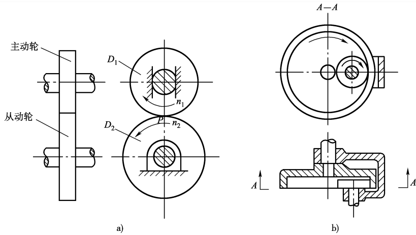
图 15-1 摩擦轮传动
