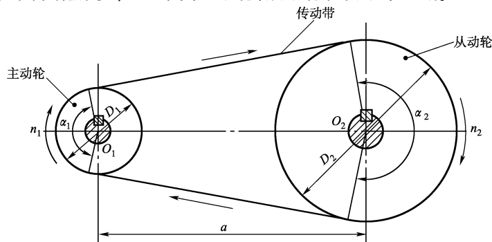
图 1-26 带传动简图
