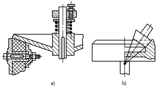
图 员圆 两轴相交的摩擦轮传动 圆外接圆锥式, 圆内接圆锥式
