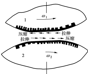
图 1.10 摩擦轮传动的弹性滑动 1—主动轮 2—从动轮
