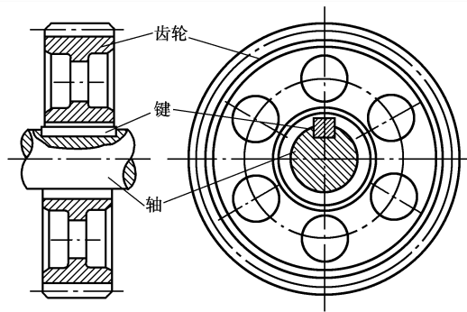
图 1-1 机构构件
