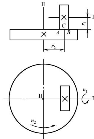
图 员圆 圆柱圆盘式摩擦轮传动
