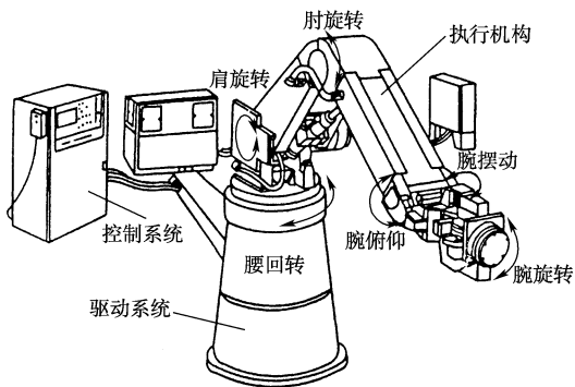
图 园 摇工业机器人
