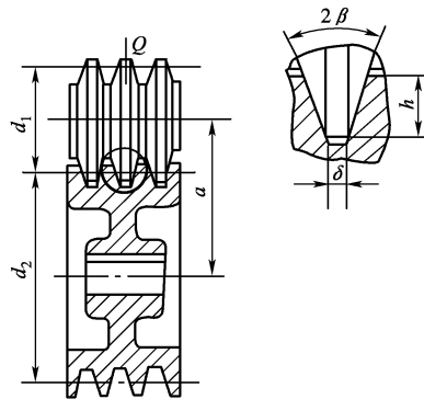
图 员圆 圆柱槽摩擦轮传动
