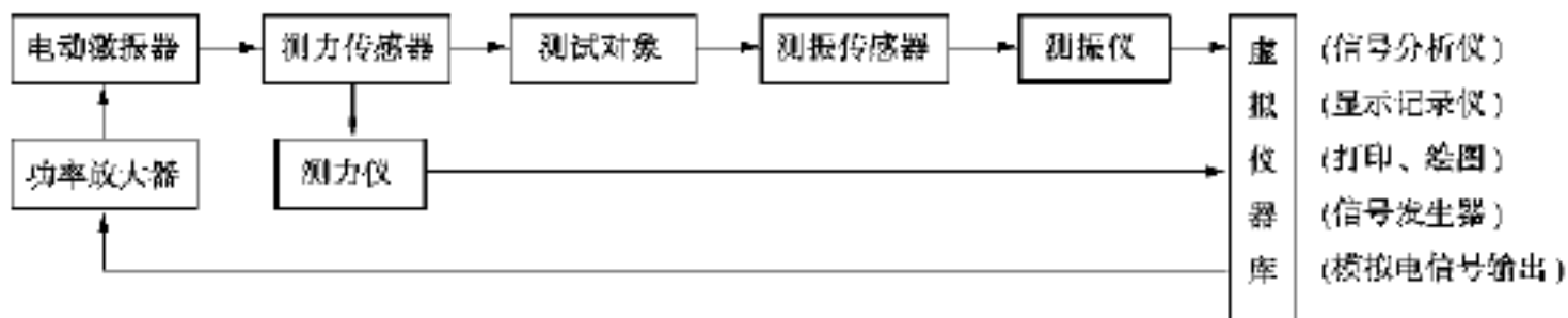
图 0.2 构建频率响应测试系统
